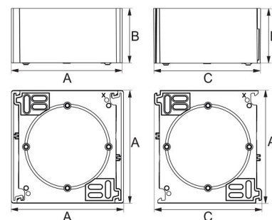
باکس های روکار (mm)
